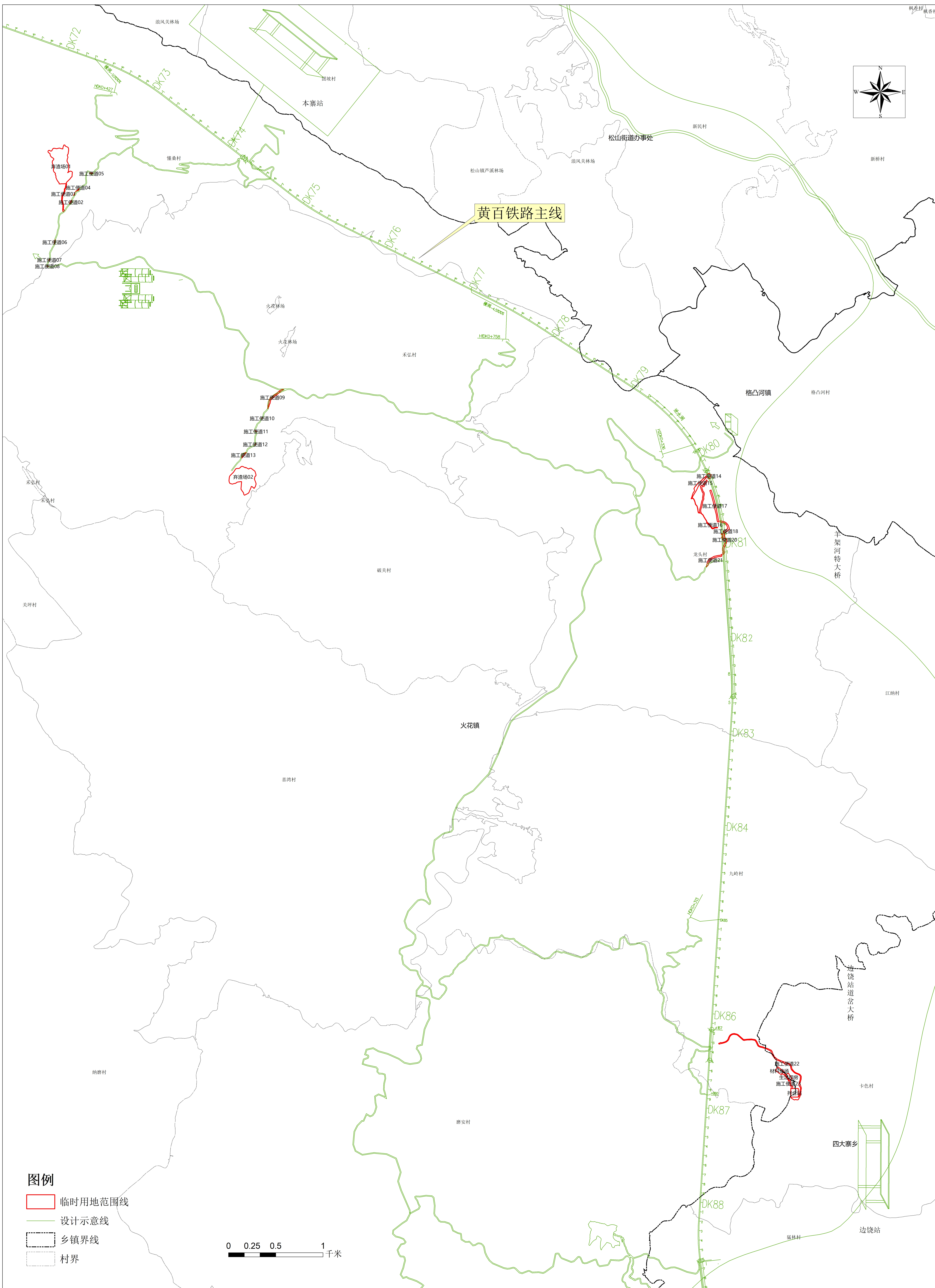
黄百铁路（贵州段）工程HBZQ-3标紫云县火花至四大寨段第二批临时用地平面布置图
